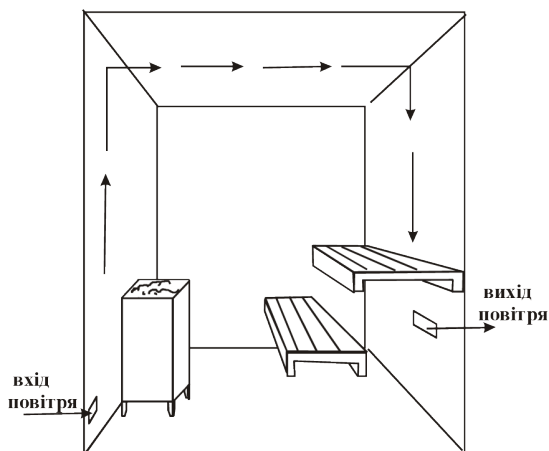
Рисунок 3 - Схема повітрообміну в парильному приміщенні
