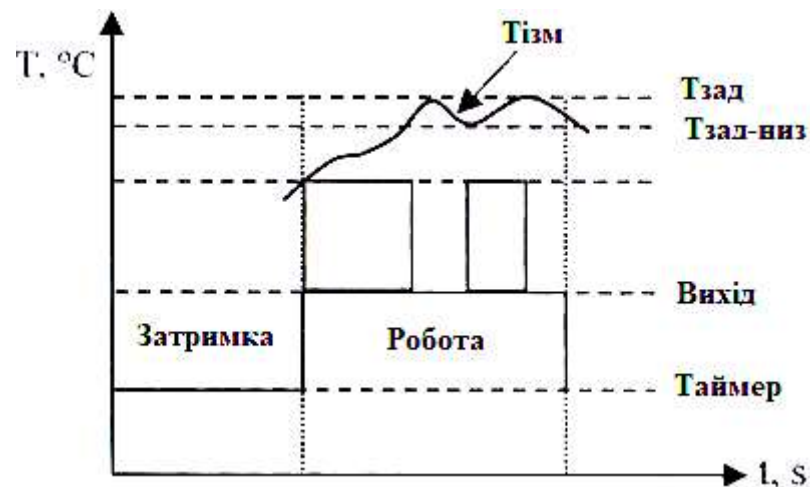
Рисунок 4. Графік роботи таймера
