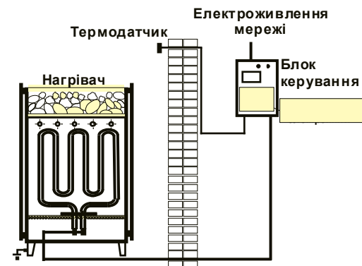
Рисунок 1 - Схема установки і підключення ЕКС
