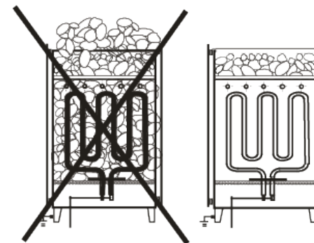
Рисунок 2 - Укладання каміння
