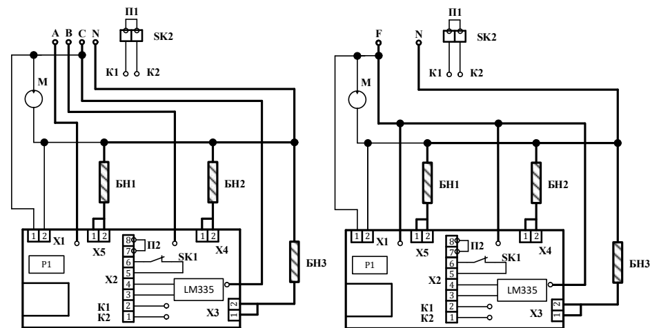
Рисунок 4 - Схема електрична принципова
