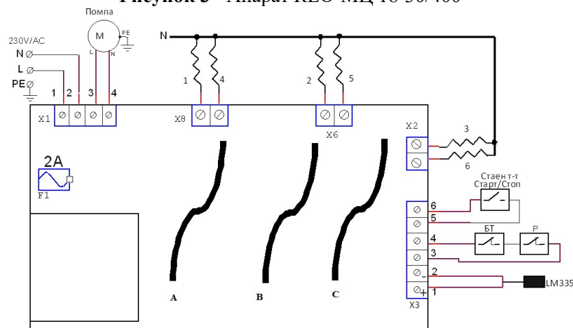
Рисунок 4 - Схема електрична принципова
